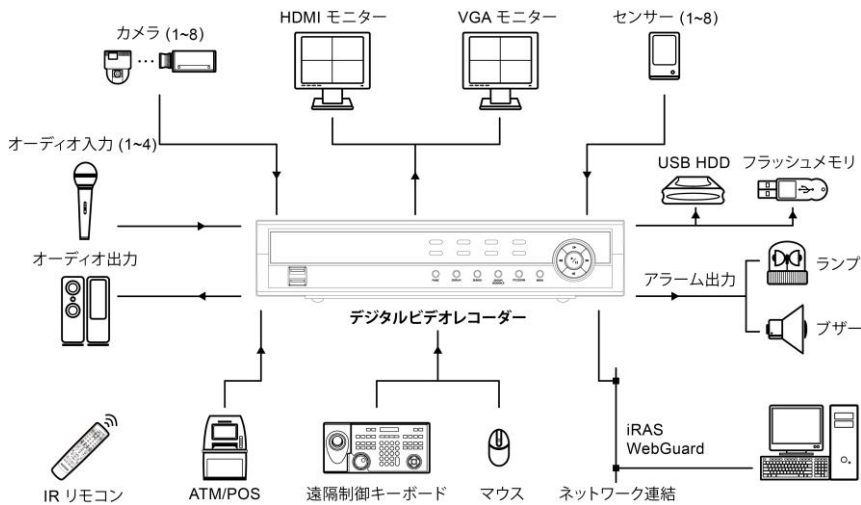
図1: サンプル構成図
