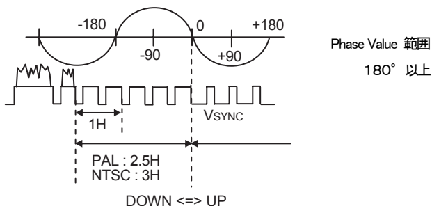
図 9-3 PHASE SHIFT
